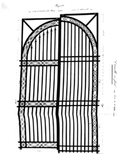
Fig. 16 - Rilievi per la riordinazione del Mercato Boario, prospetti - sono rappresentate le due metà - dei cancelli d'ingresso al mercato dal cortile della rocca e viceversa (ASCF, Miscellanea , b. 14, 1866-1886)
