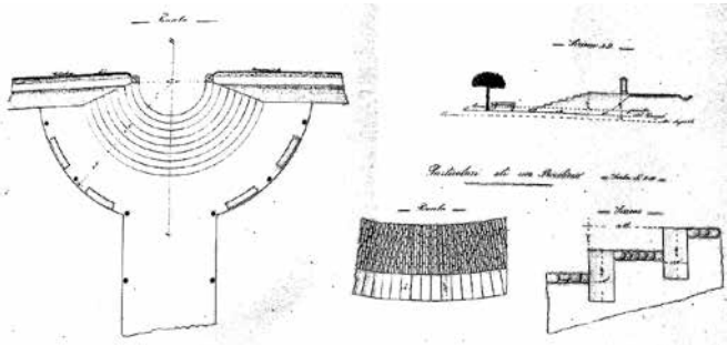
Fig. 17 - Rilievi per la riordinazione del Mercato Boario, scala con particolari di un gradino (ASCF, Miscellanea , b. 14, 1866-1886)
