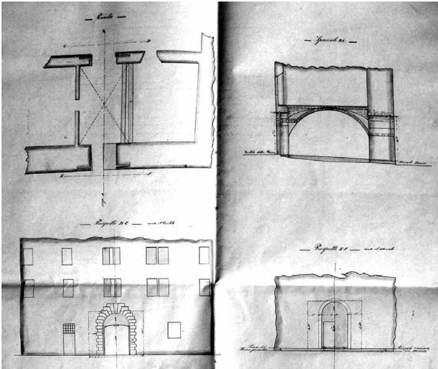
Fig. 15 - Rilievi per la riordinazione del Mercato Boario, pianta e sezione del passaggio con prospetti degli ingressi in quest'ultimo - tra Foro boario e rocca (ASCF, Miscellanea , b. 14, 1866-1886)
